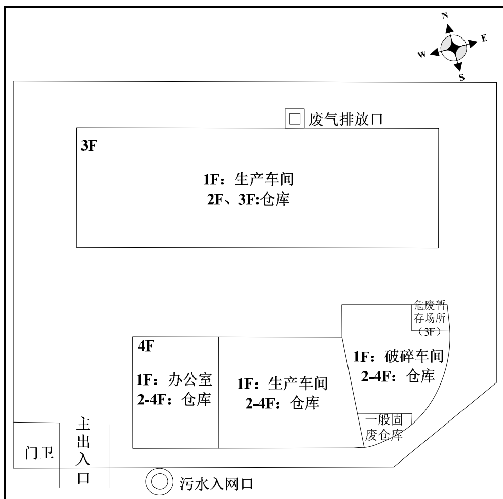
图 3-2 平面布置图
