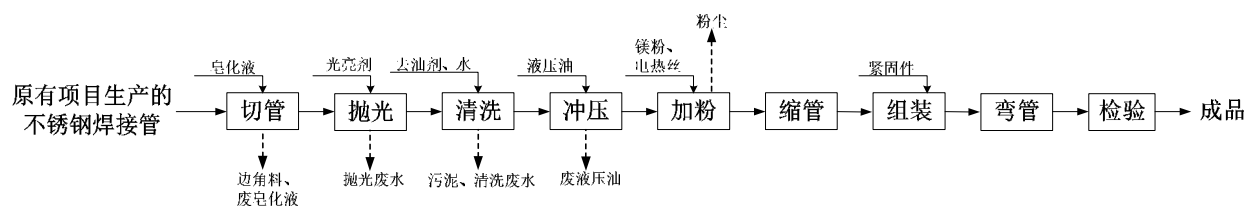
图 3-4 环评审批生产工艺流程及产污环节图
