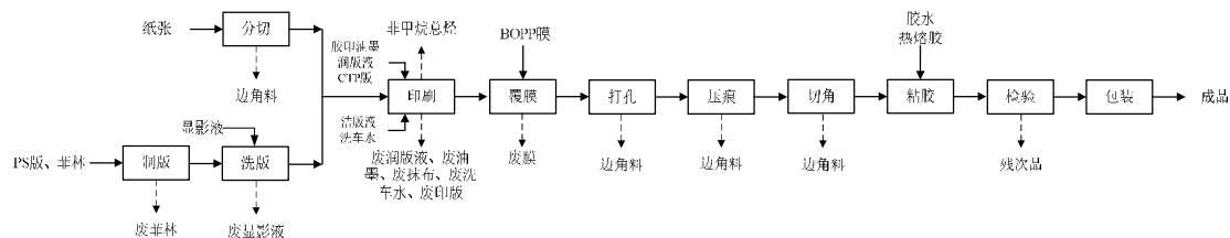
图 3-4 环评审批吊牌、彩盒生产工艺流程及产污环节图
