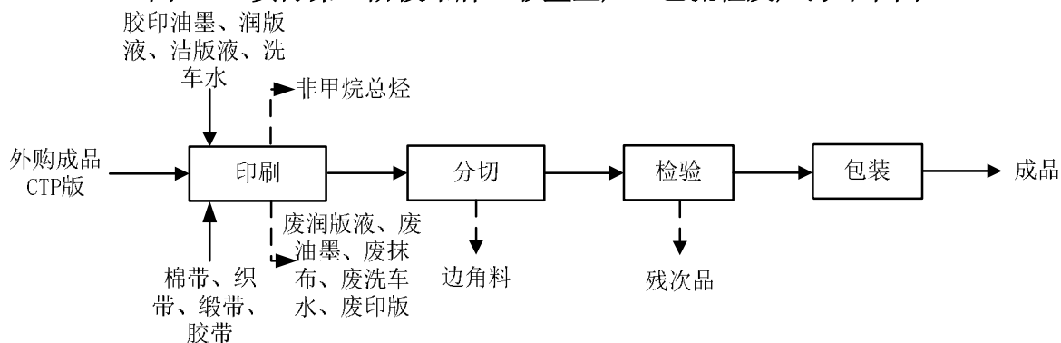
图 3-7 实际第一阶段水洗标生产工艺流程及产污环节图
