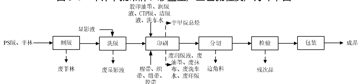
图 3-5 环评审批水洗标生产工艺流程及产污环节图
