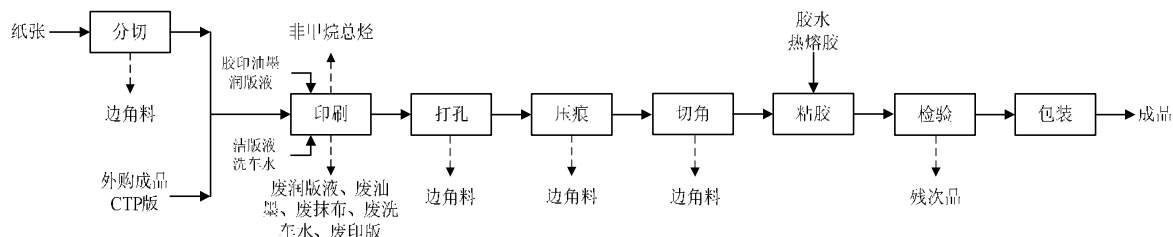
图 3-6 实际第一阶段吊牌、彩盒生产工艺流程及产污环节图
