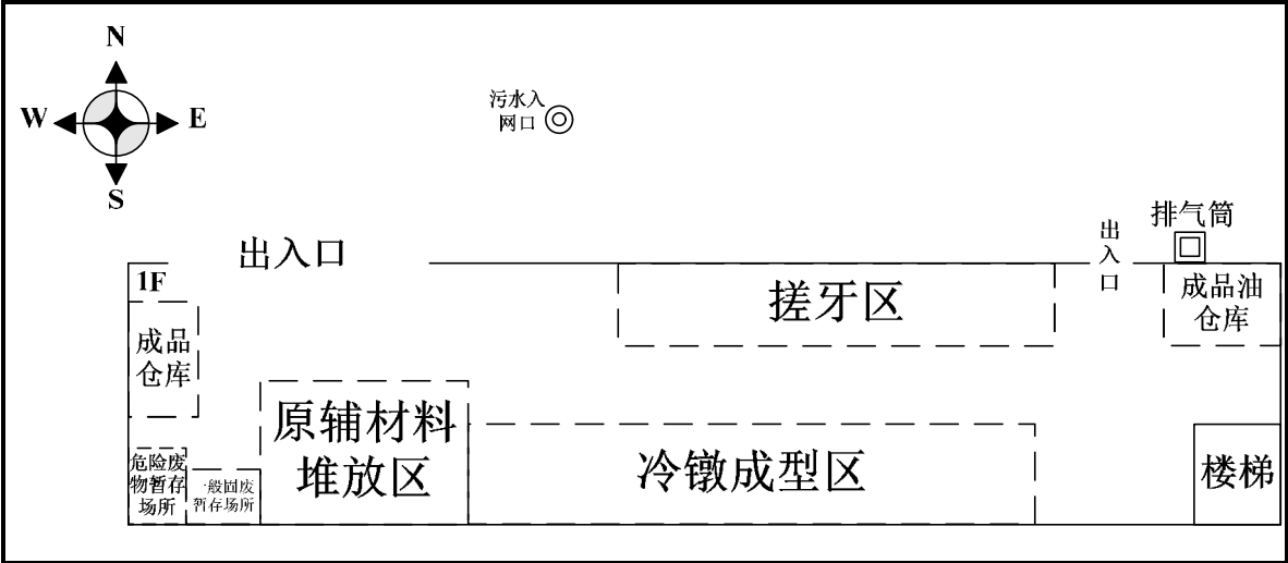
图 3-2 平面布置图
