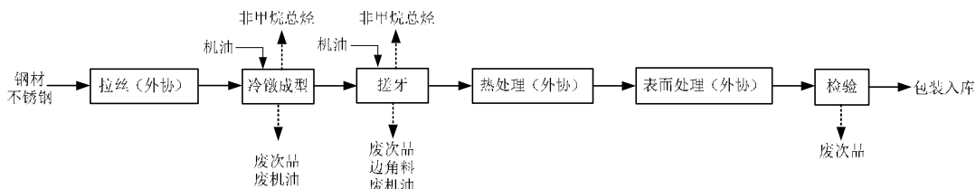
图 3-4 本项目生产工艺流程及产污环节图
