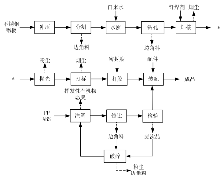
图 3-4 本项目生产工艺流程及产污环节图
