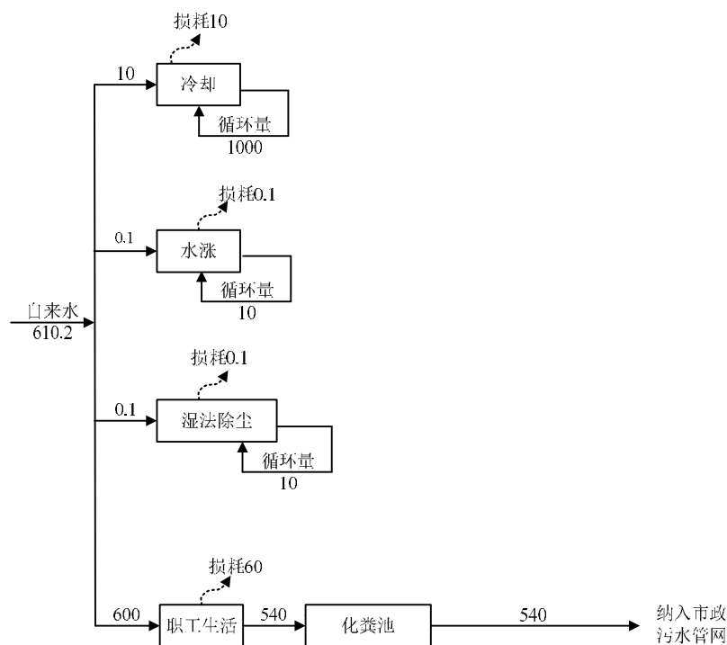
图 3-3 本项目水平衡图
