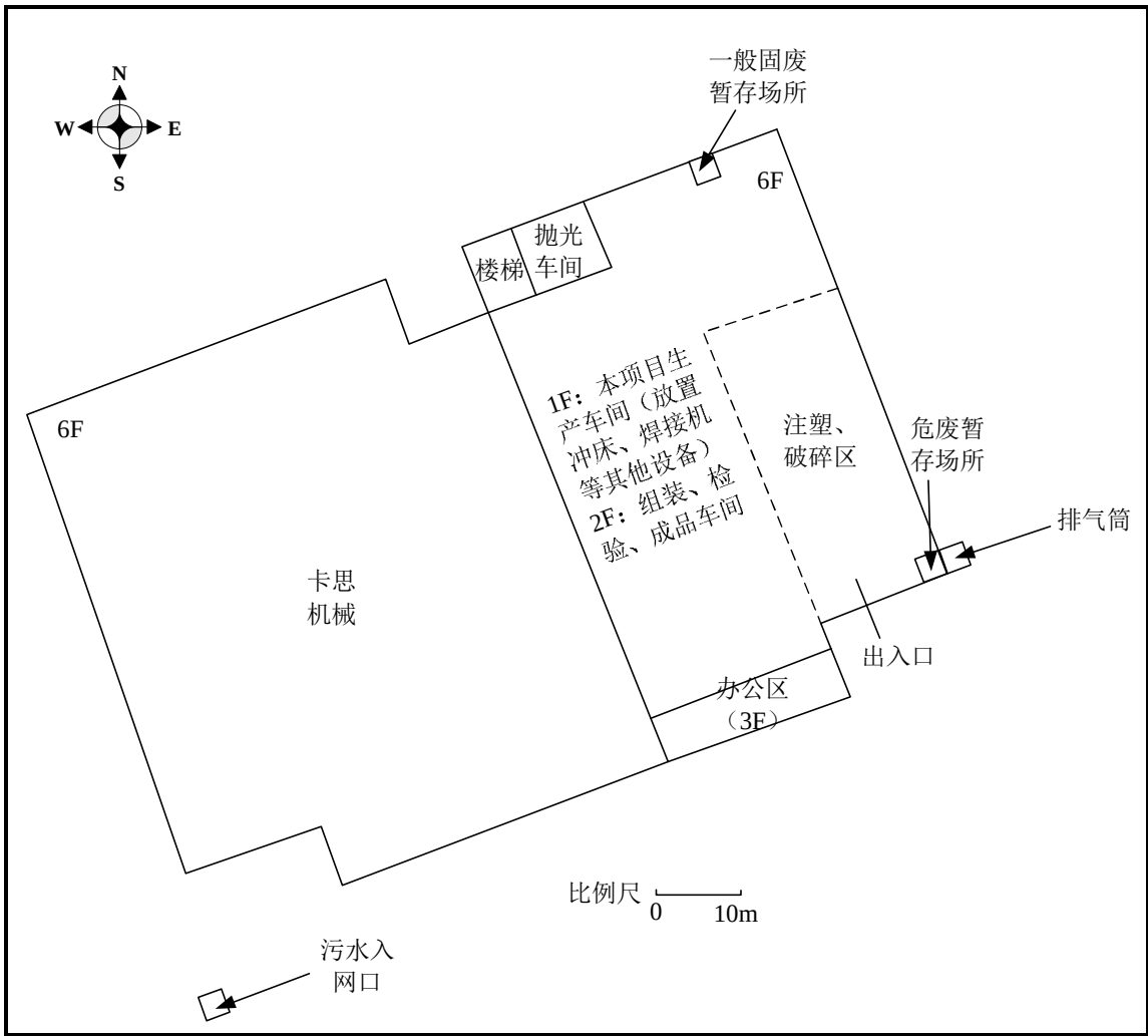
图 3-2 平面布置图
