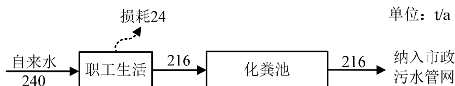
图 3-3 本项目水平衡图
