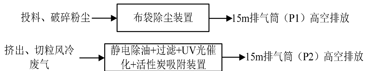
图 4-1 废气治理流程图
