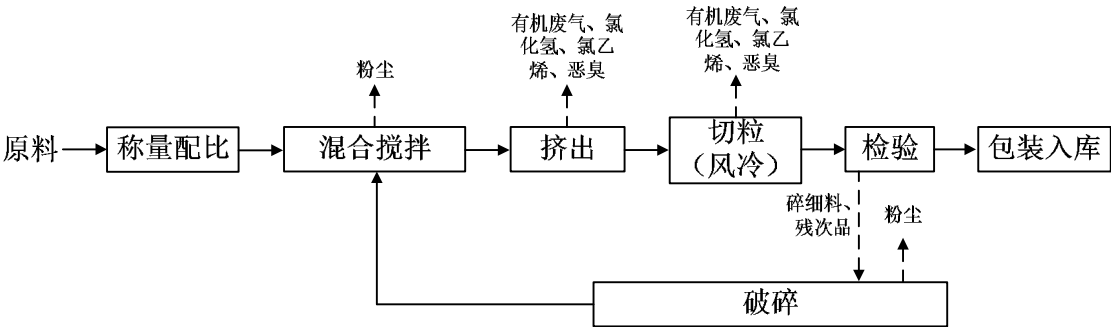
图 3-4 环评审批生产工艺流程及产污环节图
