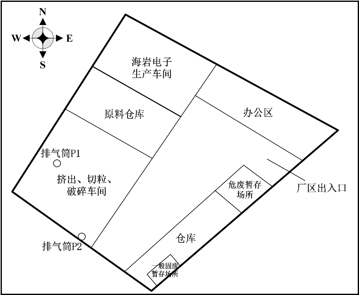
图 3-2 平面布置图
