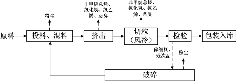
图 3-5 实际第一阶段生产工艺流程及产污环节图
