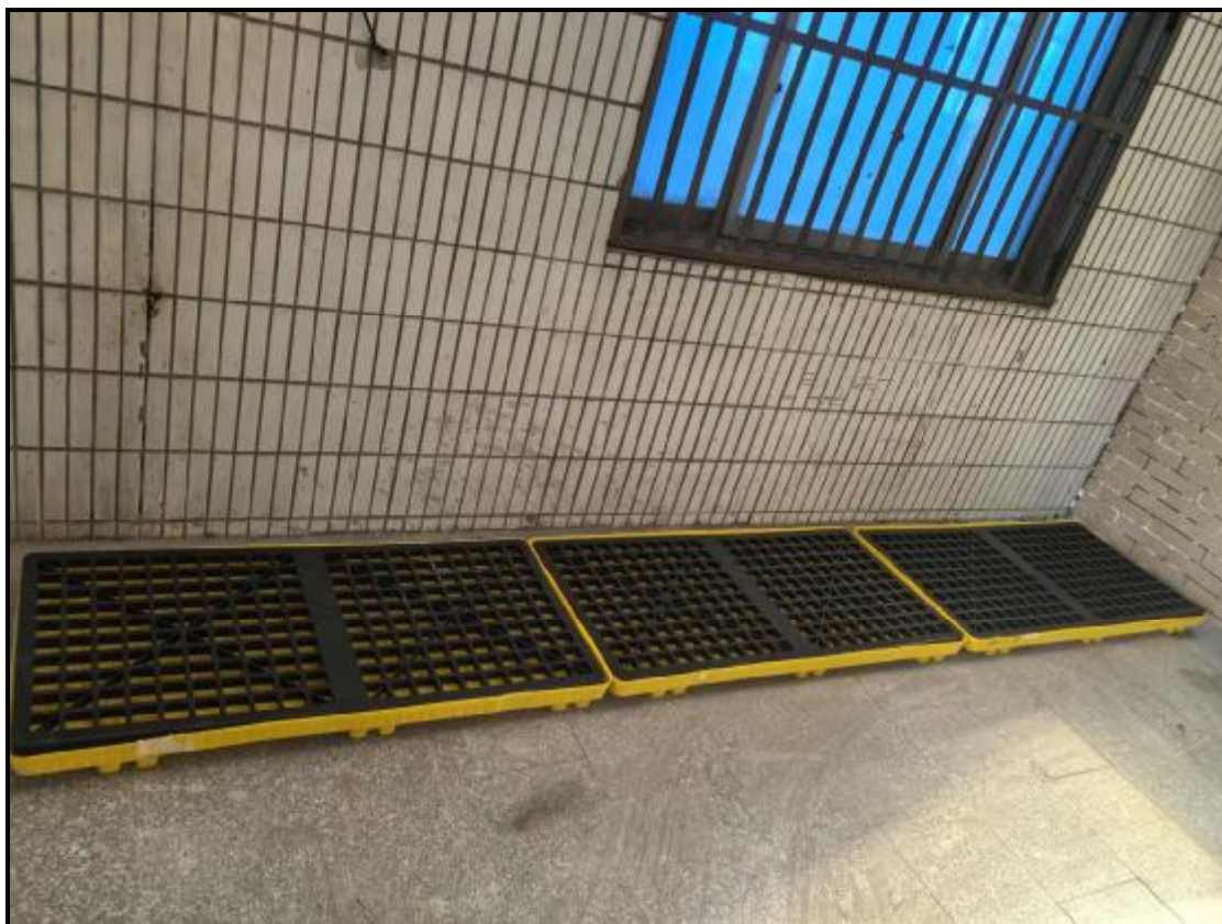
图 4-5 危废暂存场所照片（内部）
