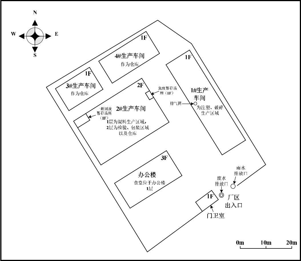
图 3-2 平面布置图
