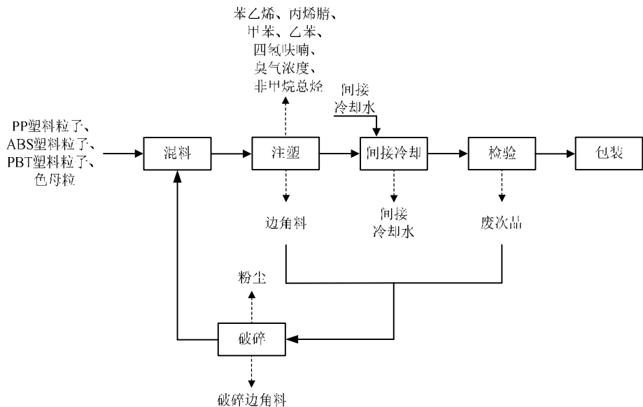
图 3-4 本项目生产工艺流程及产污环节图
