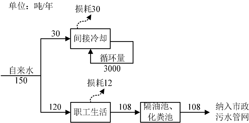
图 3-3 本项目水平衡图
