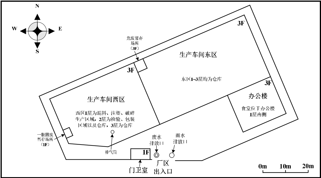
图 3-2 平面布置图
