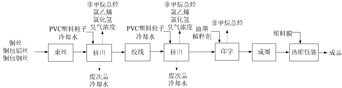
图 3-4 本项目生产工艺流程及产污环节图
