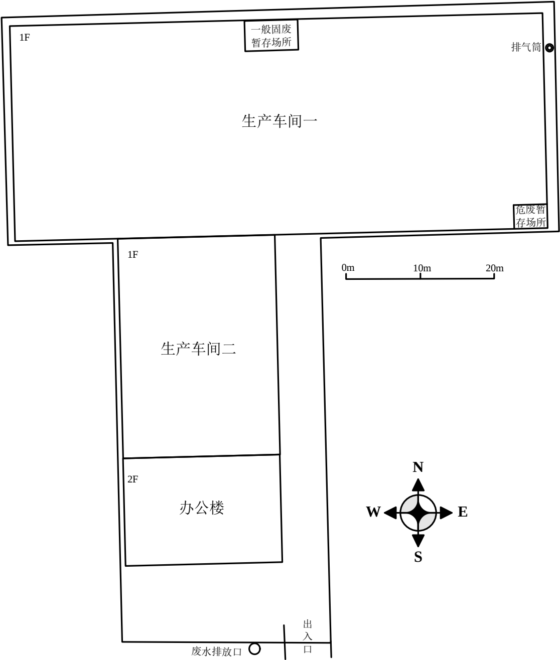
图 3-2 平面布置图
