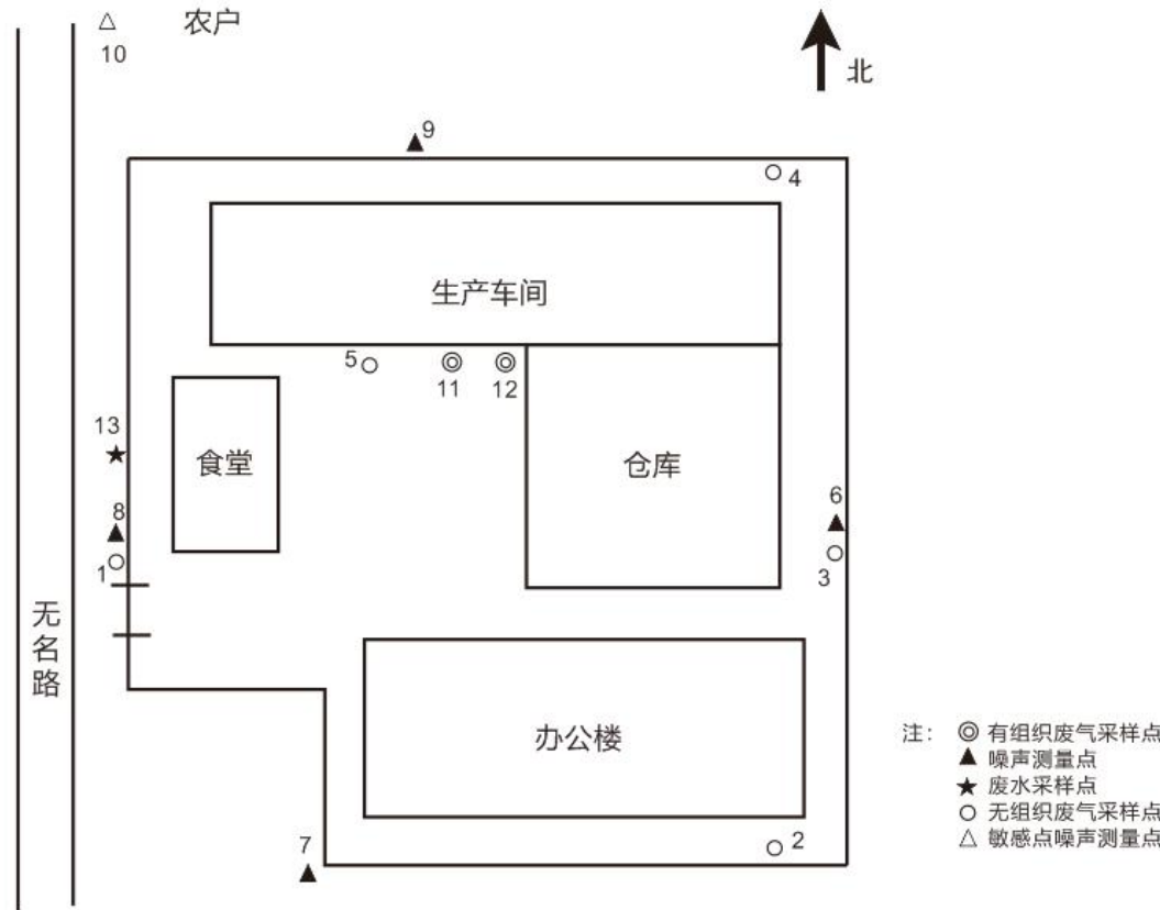
图 7-1 监测、采样点位示意图
