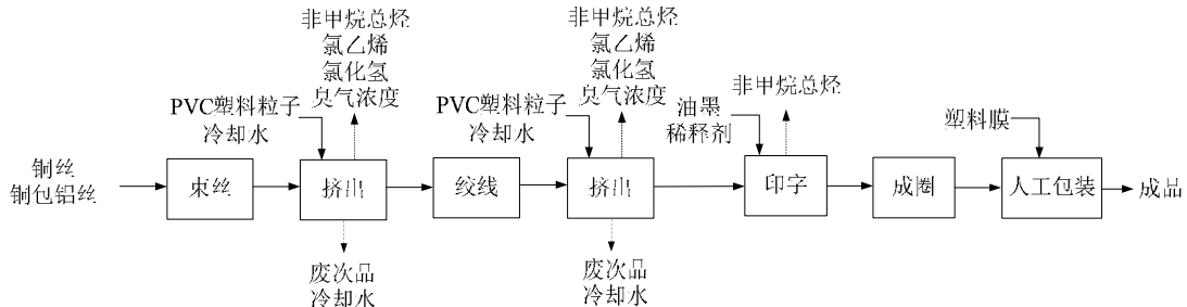
图 3-5 实际第一阶段生产工艺流程及产污环节图
