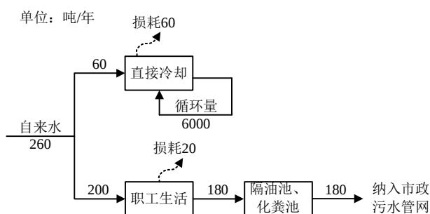
图 3-3 本项目水平衡图
