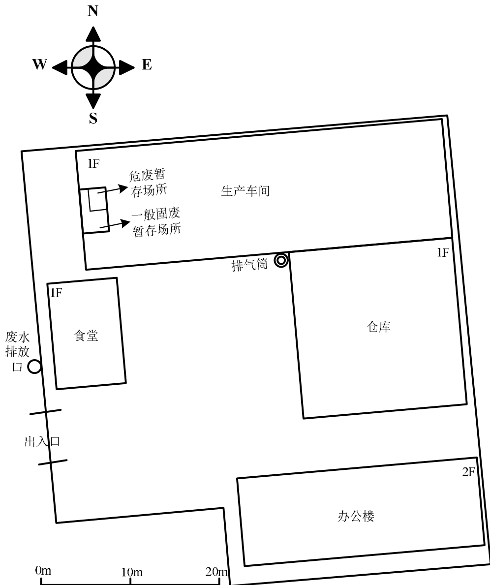
图 3-2 平面布置图
