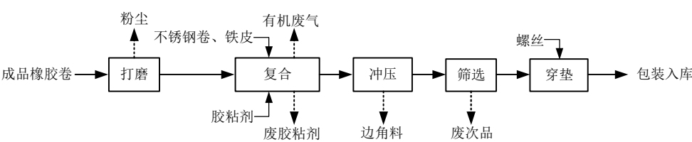
图 3-4 环评审批生产工艺流程及产污环节图
