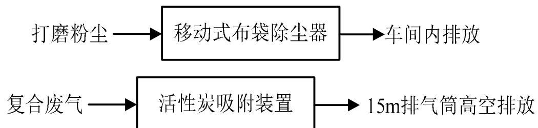
图 4-1 废气治理流程图
